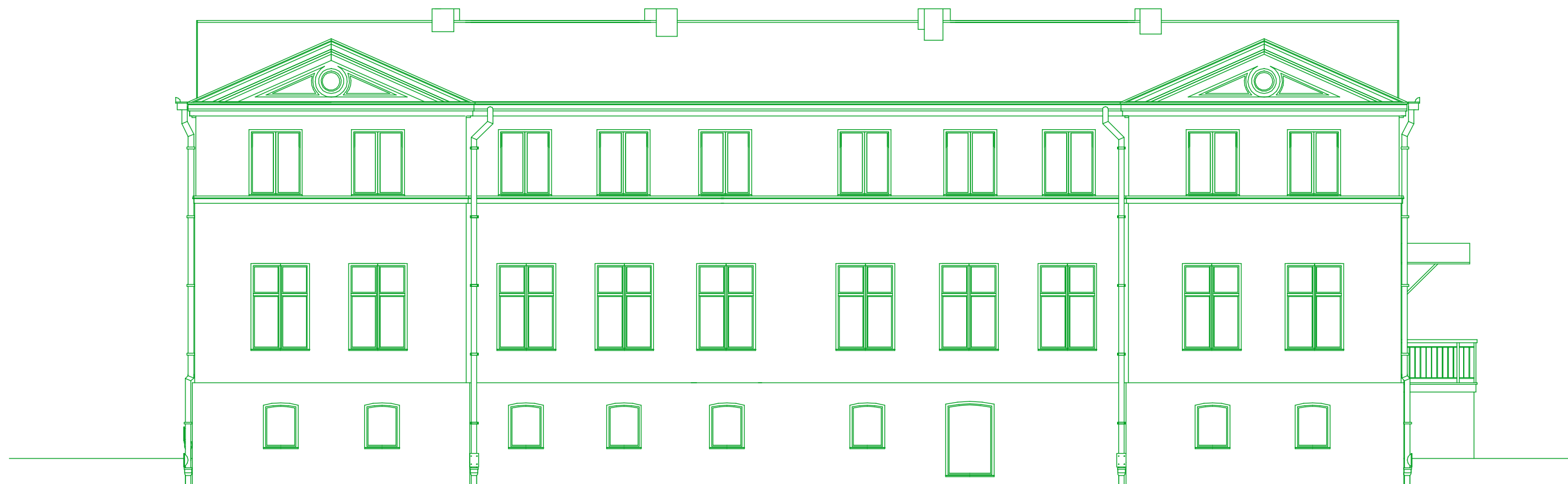
ELEWACJA ZACHODNIA
